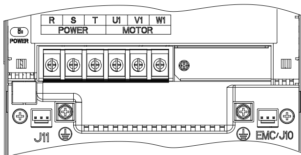
Рис. 3-7 Схема клемм основной цепи 11–15кВт
