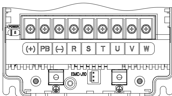
Рис. 3-6 Схема клемм основной цепи 7.5кВт
