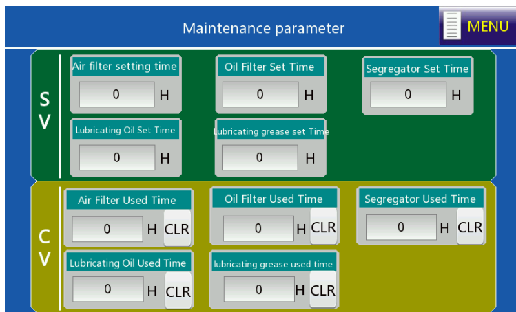
Рис. 4-11 Интерфейс параметров обслуживания
