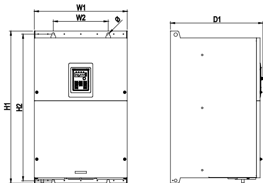
Рис. 7-4 Размеры для настенного монтажа 90кВт–110кВт
